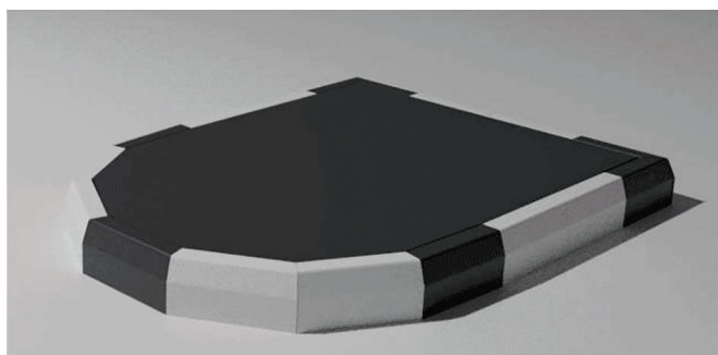
Рисунок Б.12 - Пример устройства защитных элементов на улицах с двумя полосами движения при помощи делиниаторов с дорожными пластинами
