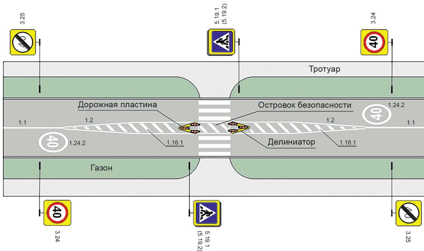
Рисунок Б.14 - Пример обустройства пешеходного перехода сигнальными пластинами на улицах с четырьмя полосами движения
