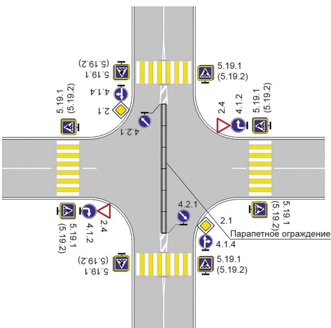
г) Перекрытие сквозного движения при помощи парапетного ограждения
