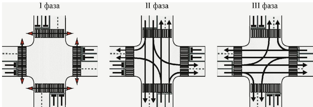
Рисунок 14. Пример светофорного регулирования на пересечении автомобильных дорог с выделением пешеходной фазы
