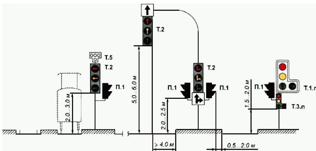
Рисунок 5. Требования к установке светофоров
