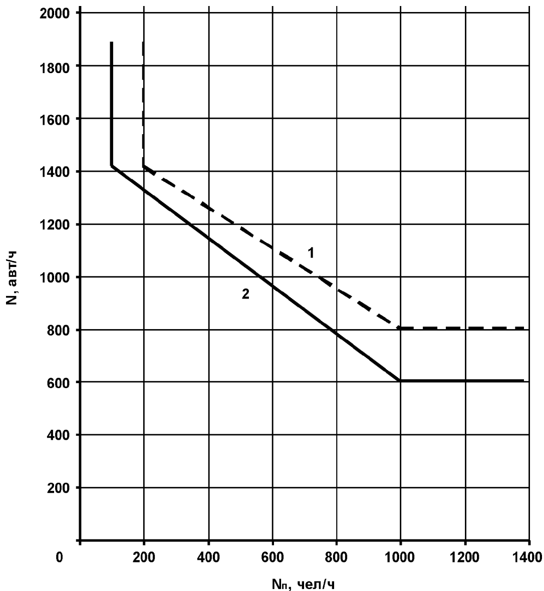
Рисунок 19. График для определения необходимости установки пешеходных светофоров вызывного действия на пешеходных переходах 1 - с островком безопасности; 2 - без островка безопасности; N - интенсивность движения транспортных средств; N_{II} - интенсивность пешеходного движения
