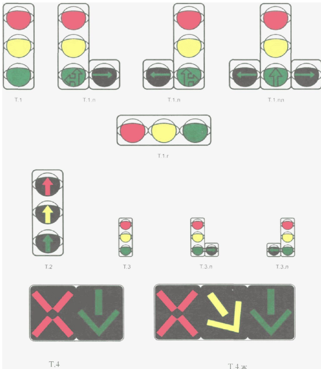
Рисунок 4а. Типы и исполнение транспортных светофоров
