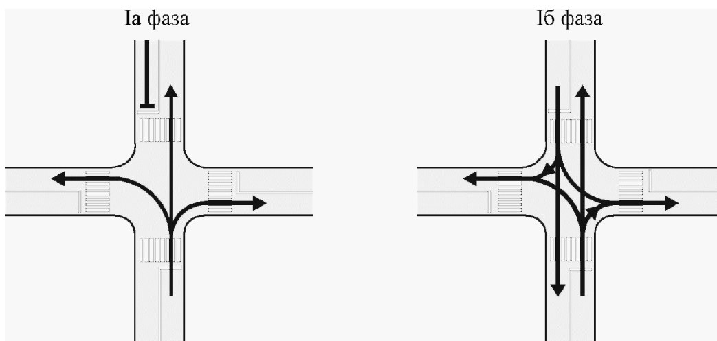
Рисунок 11. Не рекомендуемая схема организации движения
