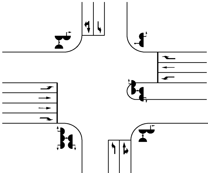
Рисунок 3. Пример расположения в плане транспортных светофоров
