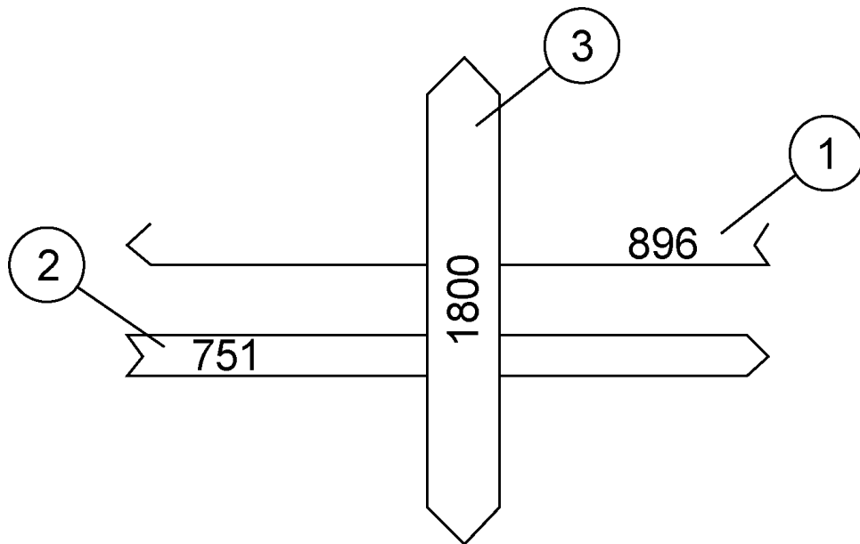
Рисунок Б.7. Картограмма интенсивностей (ед./ч, чел./ч)
