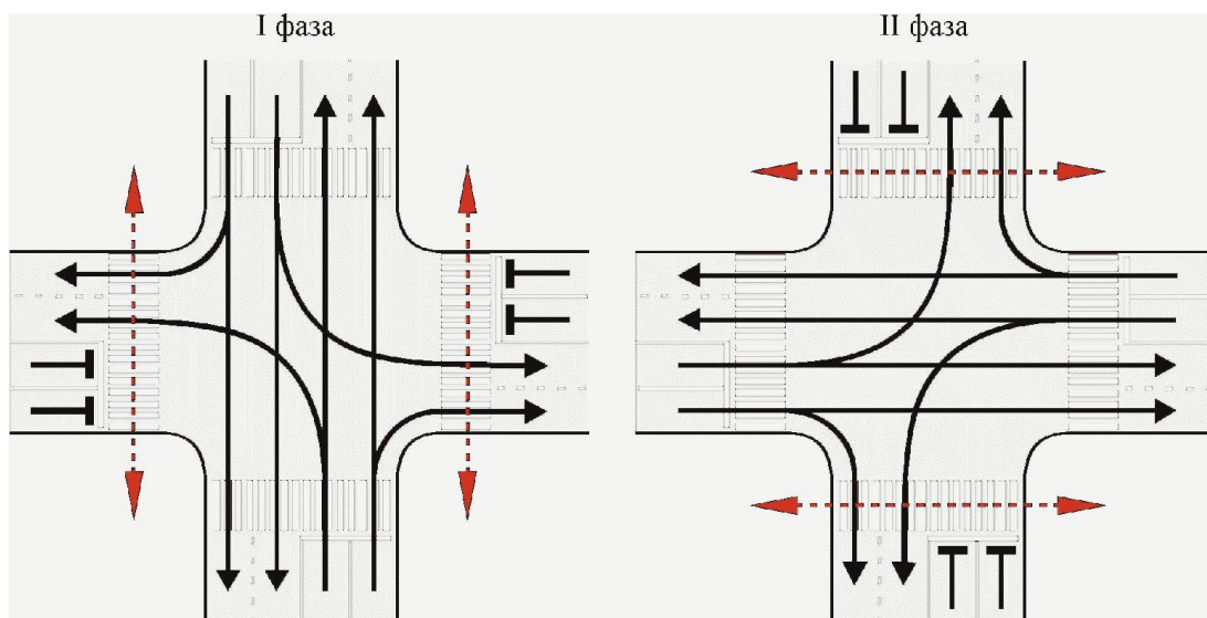
Рисунок 9. Пример двухфазного светофорного регулирования
