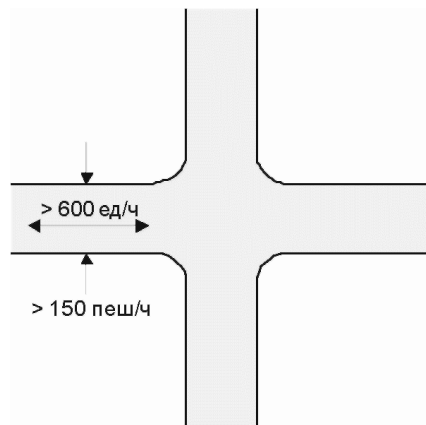
Рисунок 2. Условие N 1 для введения светофорного регулирования
