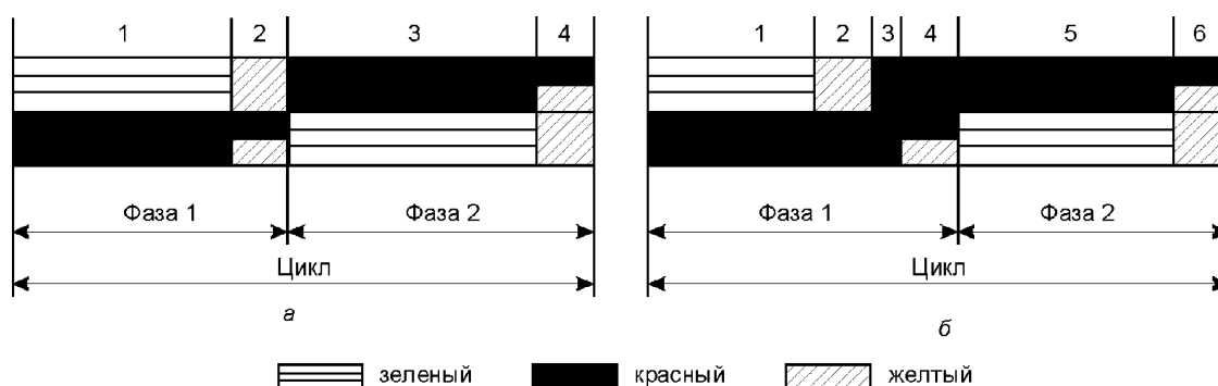
Рисунок 7. Структура светофорного цикла:
