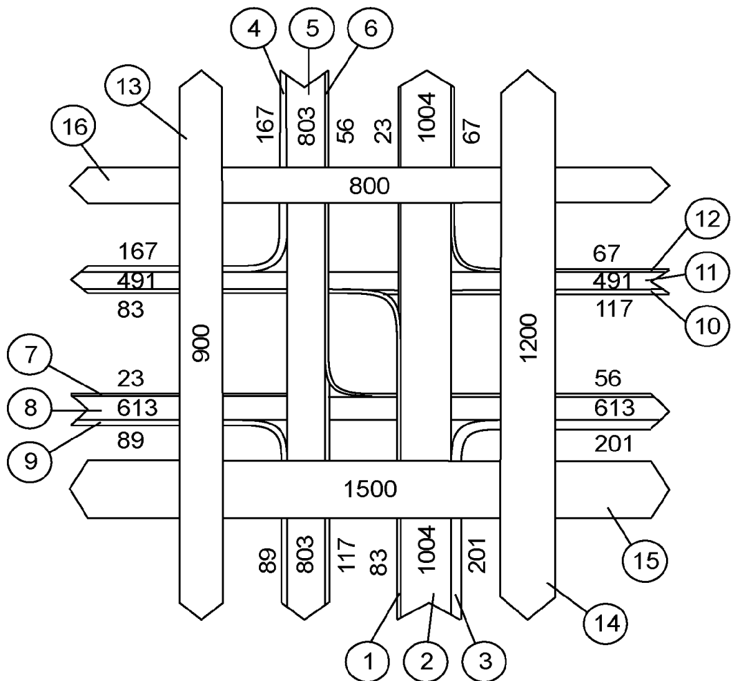
Рисунок Б.4. Картограмма интенсивностей (ед./ч, чел./ч)
