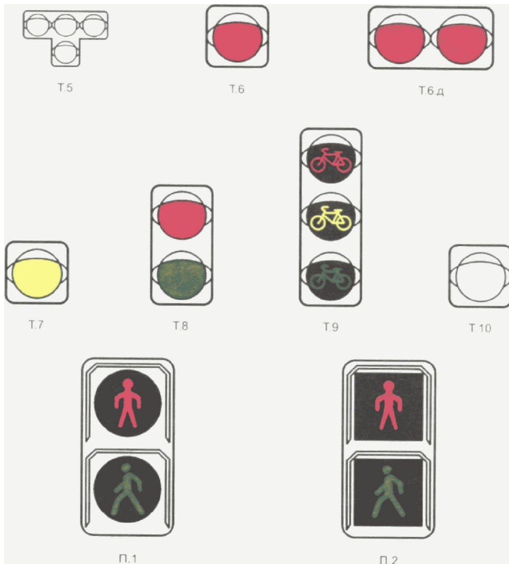
Рисунок 46. Типы и исполнение транспортных и пешеходных светофоров
