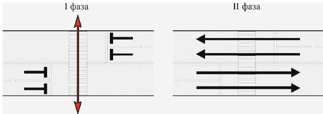
Рисунок Б.8. Пофазный разъезд транспортных и пешеходных потоков
