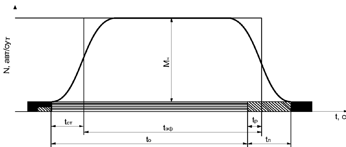
Рисунок 1. Эффективная длительность фазы регулирования
