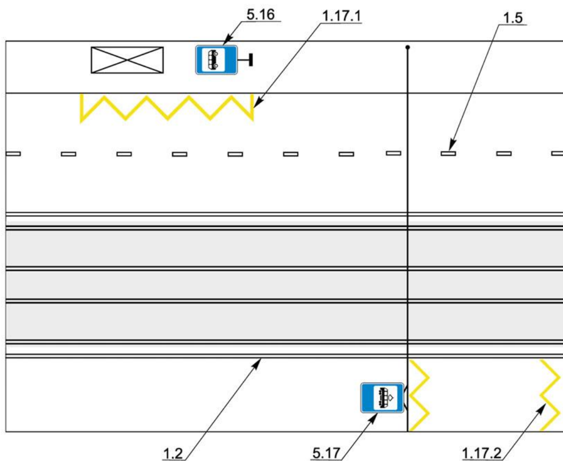
Рисунок В.15 - Пример нанесения разметки 1.17.1 и 1.17.2
