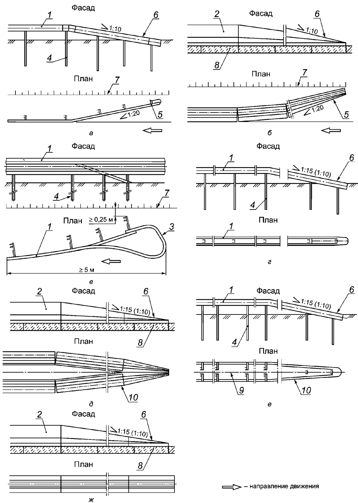
Рисунок В.29 - Примеры установки дорожных ограждений
