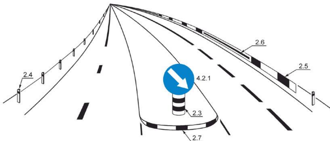
Рисунок В.24 - Пример нанесения разметки 2.3 - 2.7
