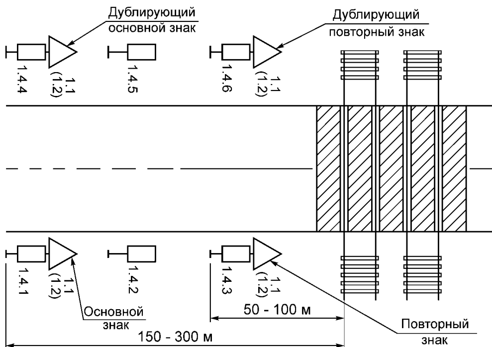
Рисунок В.3 - Размещение знаков 1.4.1 - 1.4.6
