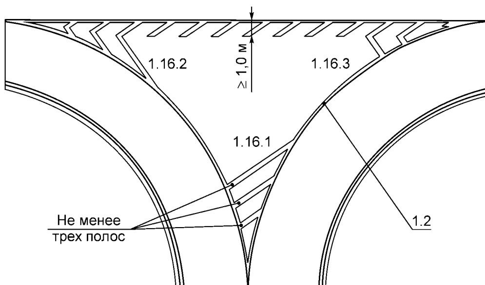
Рисунок В.12 - Пример нанесения разметки 1.16.1 - 1.16.3
