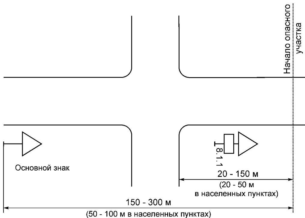
Рисунок В.1 - Типовое размещение знаков в поперечном профиле дороги
