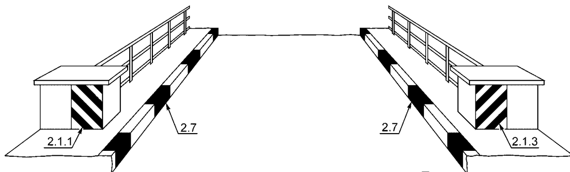
Рисунок В.23 - Пример нанесения разметки 2.1.1, 2.1.3 и 2.7
