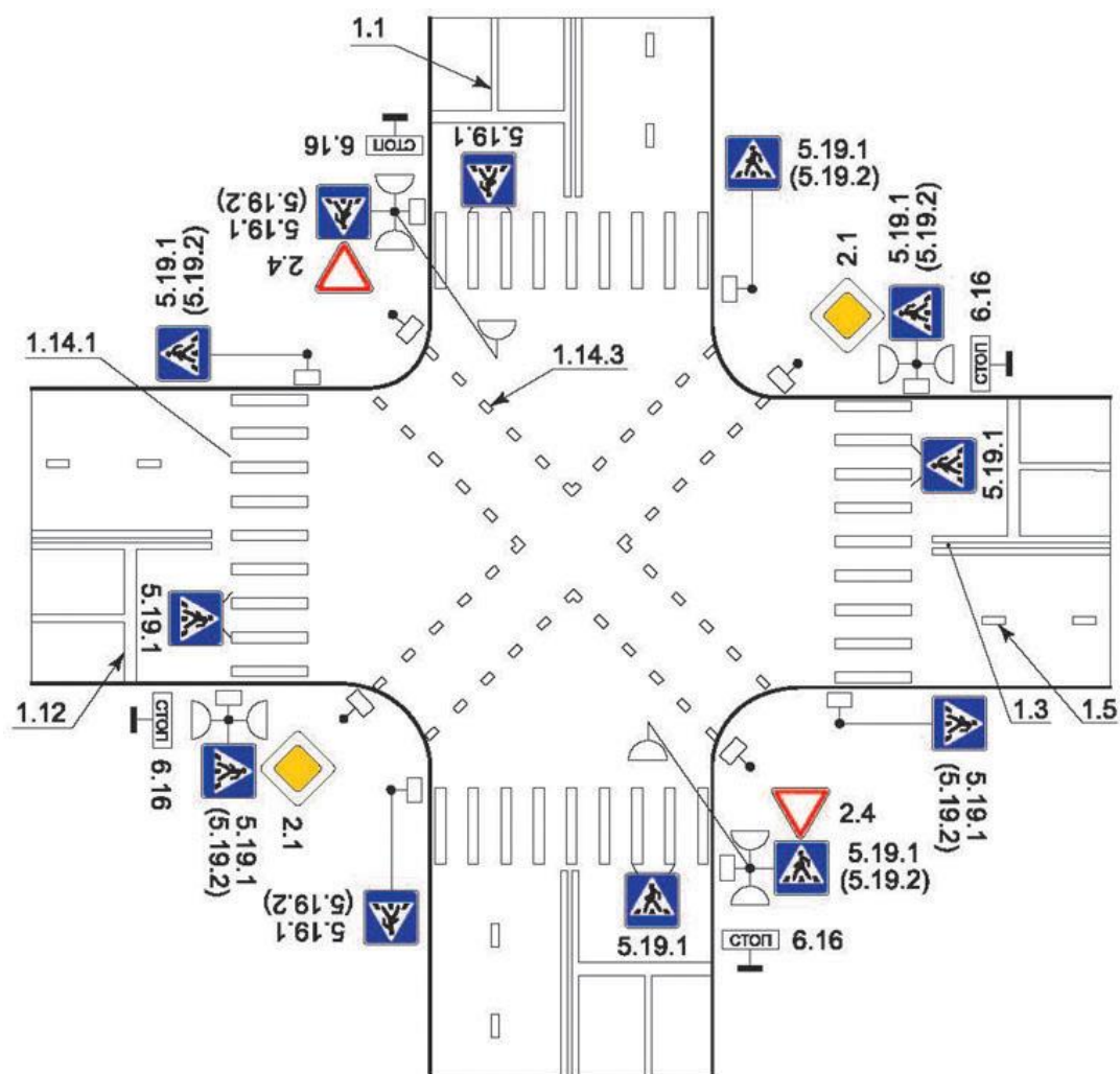
Рисунок В.19 - Пример нанесения диагонального пешеходного перехода
